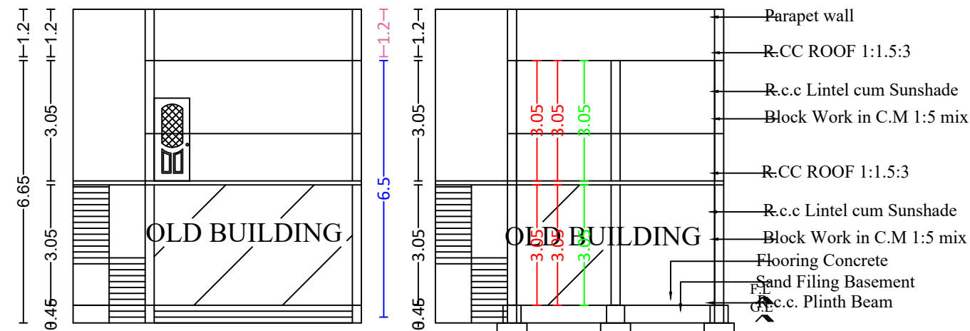
ELEVATION
