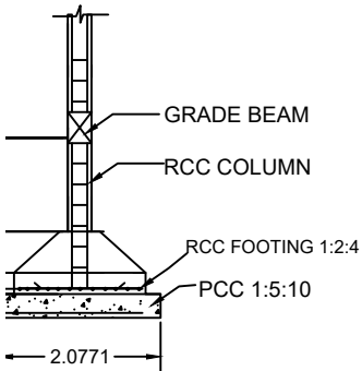
SECTION ON - BB (N.T.S)
