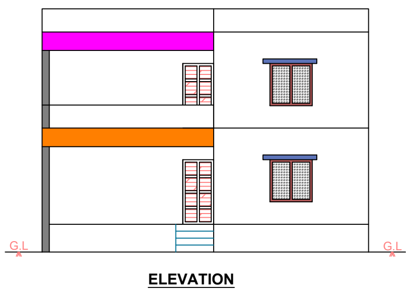
ELEVATION
