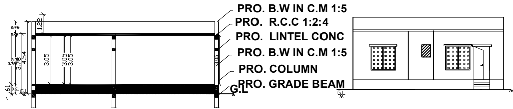
ELEVATION
