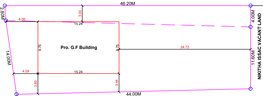
SITE PLAN (SCALE 1:200)
