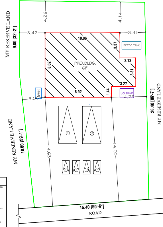
SITE PLAN 1:100
