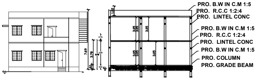
ELEVATION
