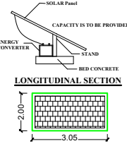
LONGITUDINAL SECTION
