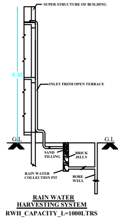
LONGITUDINAL SECTION
