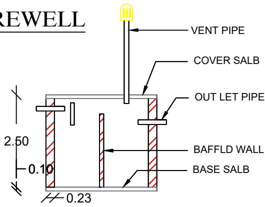
SECTION ON X - Y
