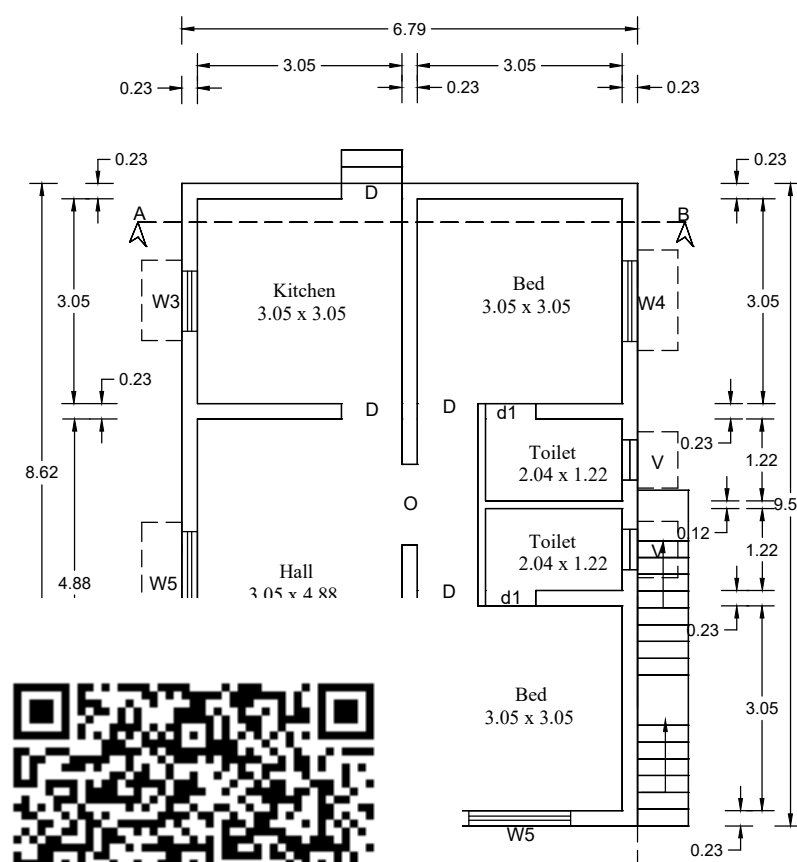
OOR PLAN
