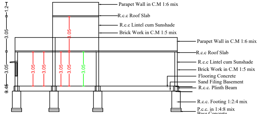
SECTION A-B
