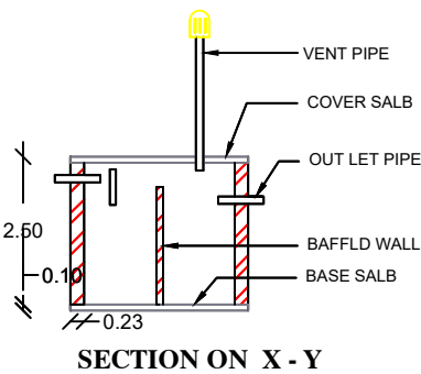
SECTION ON X - Y
