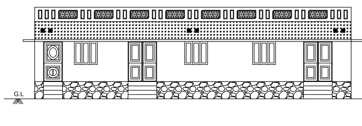
ELEVATION
