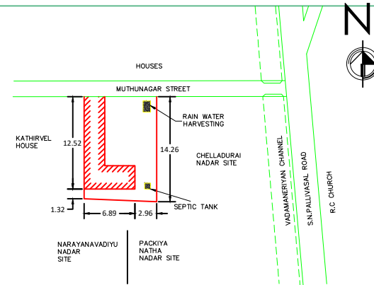
SITE PLAN (SCALE 1:400)
