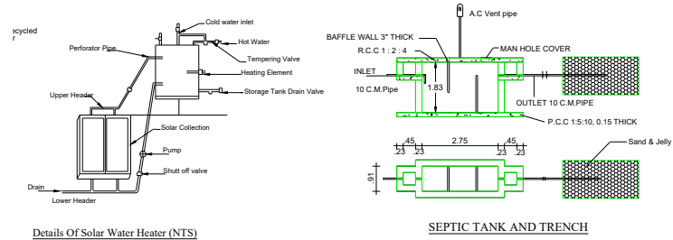
Details Of Solar Water Heater (N.T.S.)
