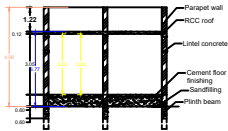
SECTION - AB
