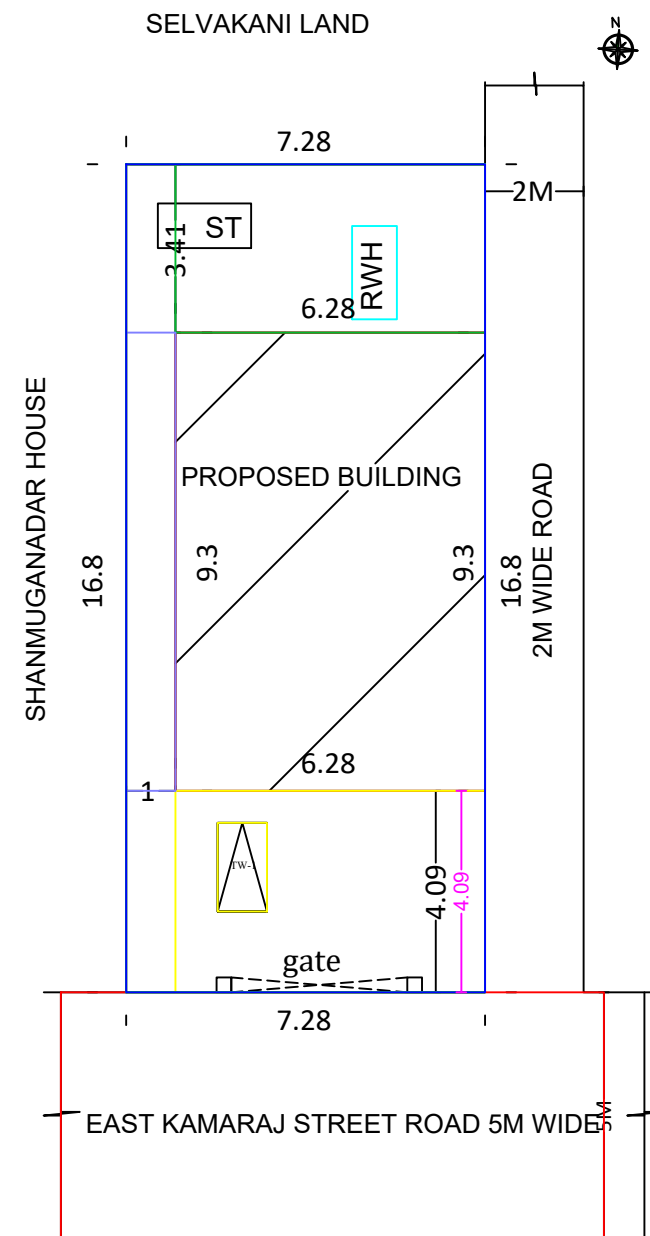
SITE PLAN 1:100 SCALE
