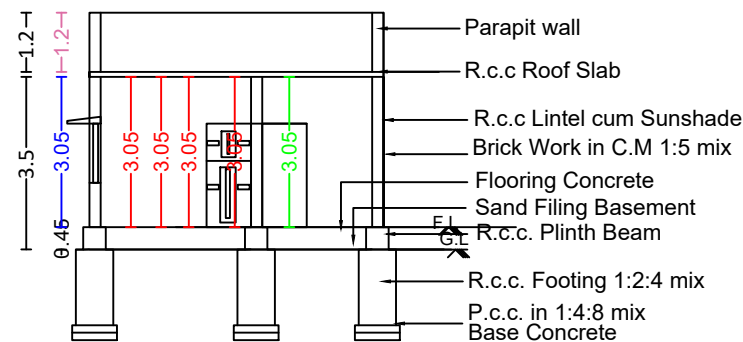
SECTION A-B
