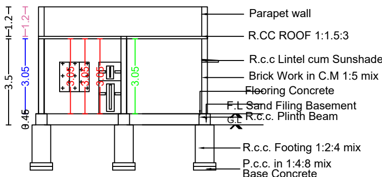
SECTION A-B
