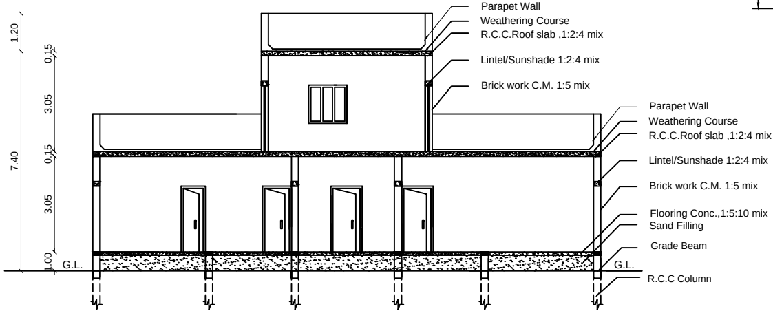
SECTION A-B
