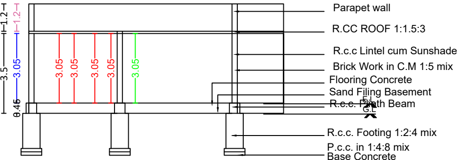
SECTION A-B
