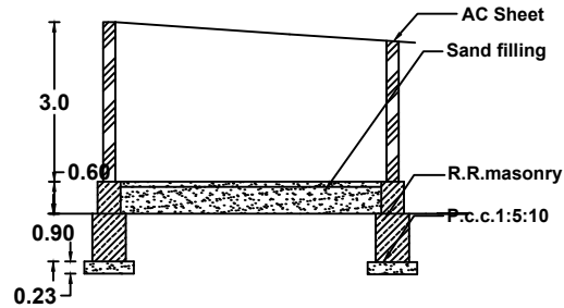
SECTION - AB
