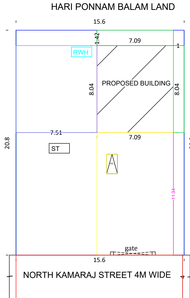
SITE PLAN 1:100 SCALE
