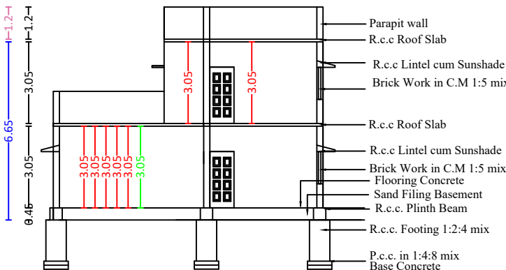
SECTION A-B
