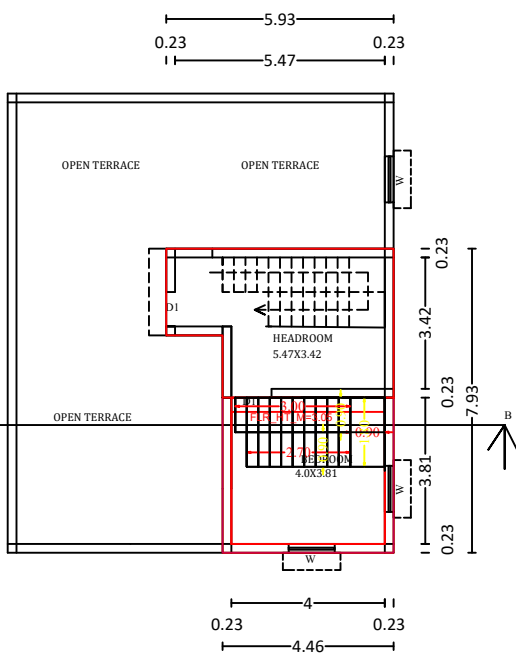
F.F. PLAN
