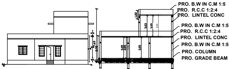
ELEVATION
