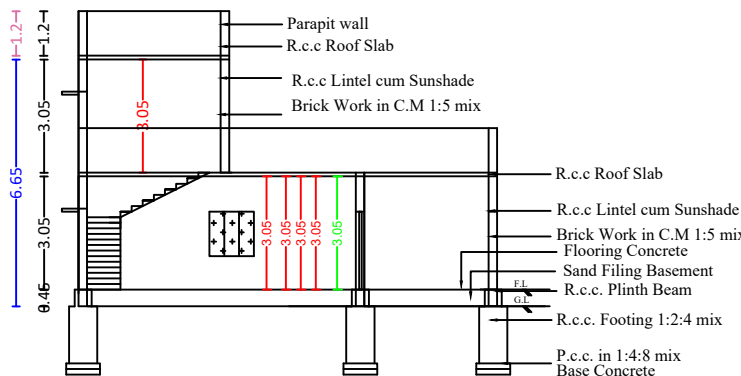
SECTION A-B
