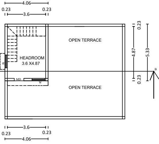
F.F. PLAN
