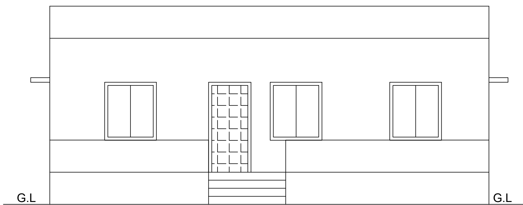
ELEVATION
