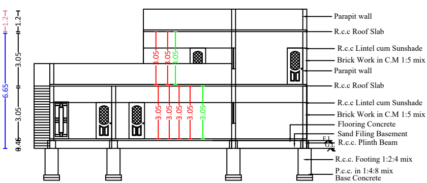
SECTION A-B
