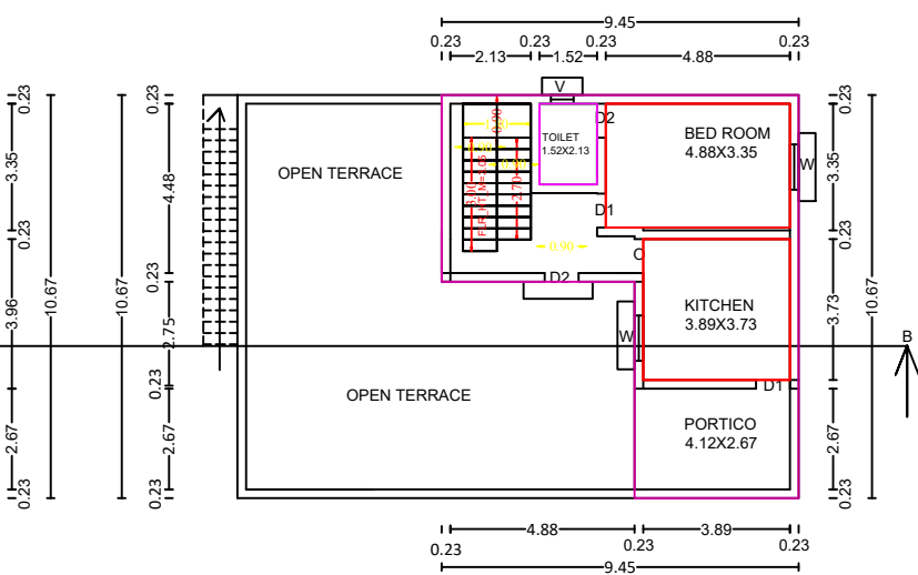
F.F.PLAN
