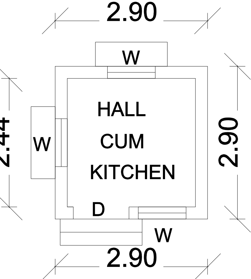
G.F PLAN
