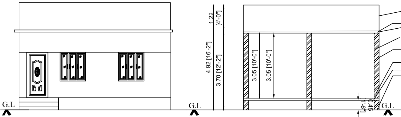
ELEVATION
