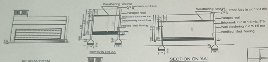
ELEVATION
