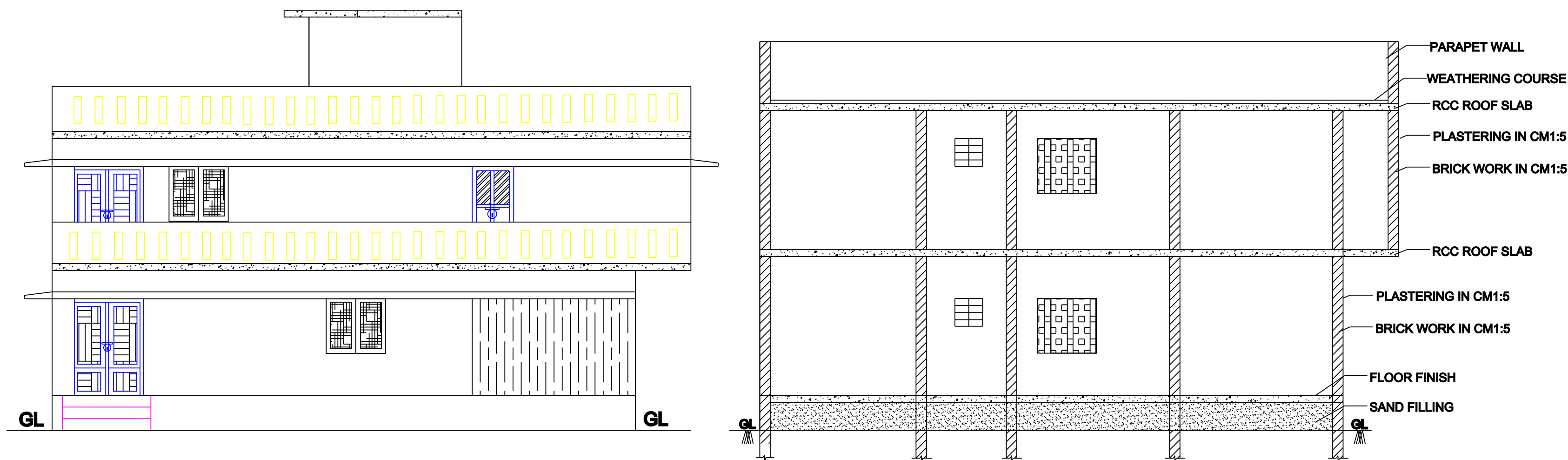
ELEVATION
