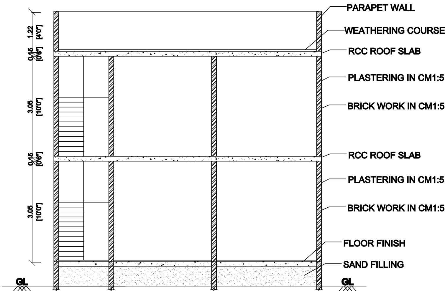
SECTION - AA' - BB'
