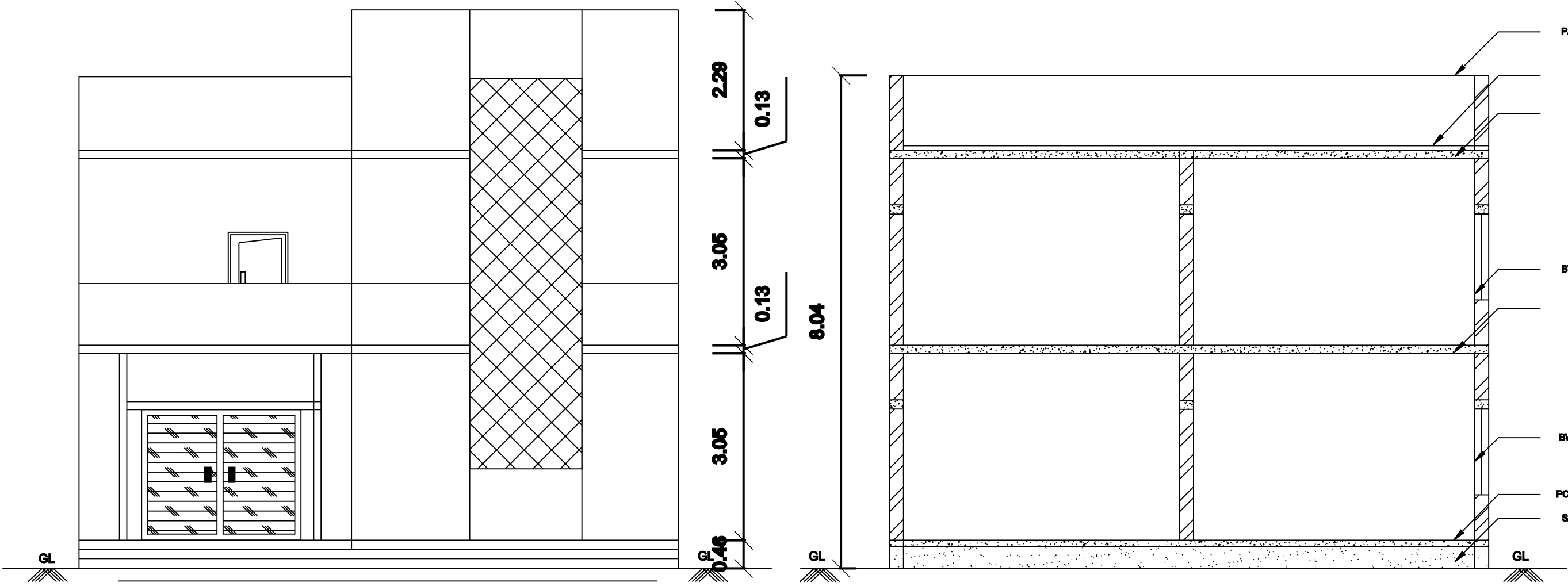
ELEVATION
