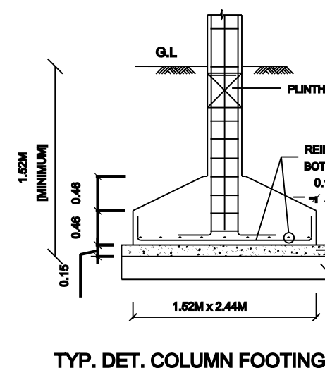
TYP. DET. COLUMN FOOTING
