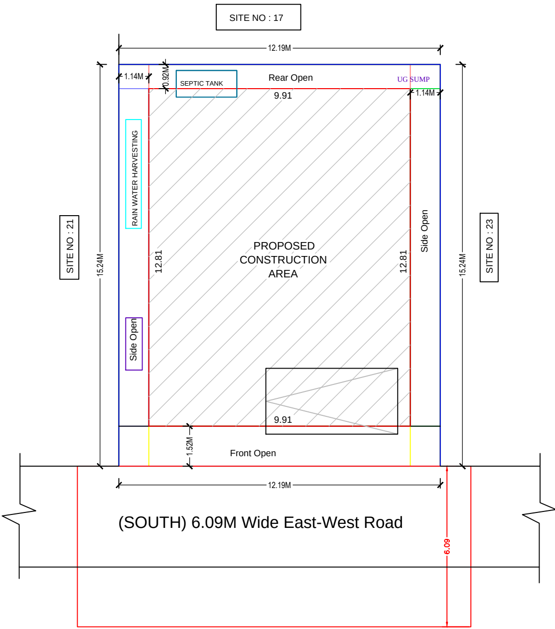
SITE PLAN-1:100
