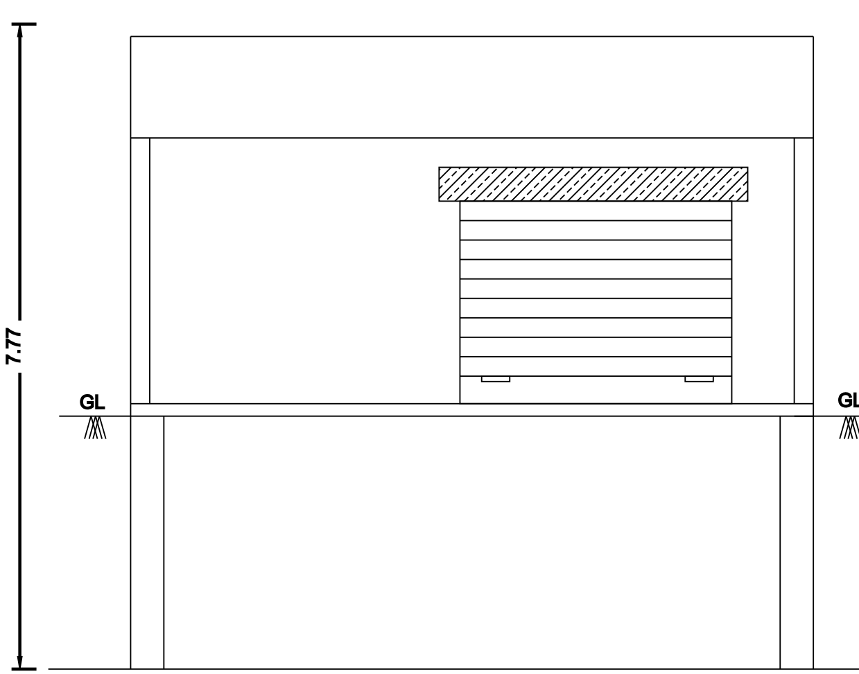
ELEVATION
