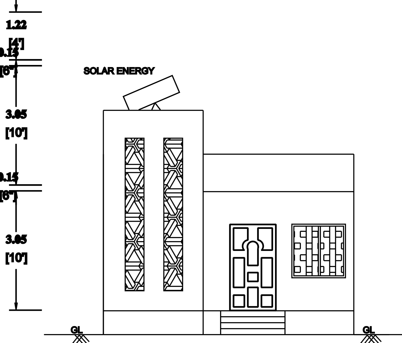
ELEVATION
