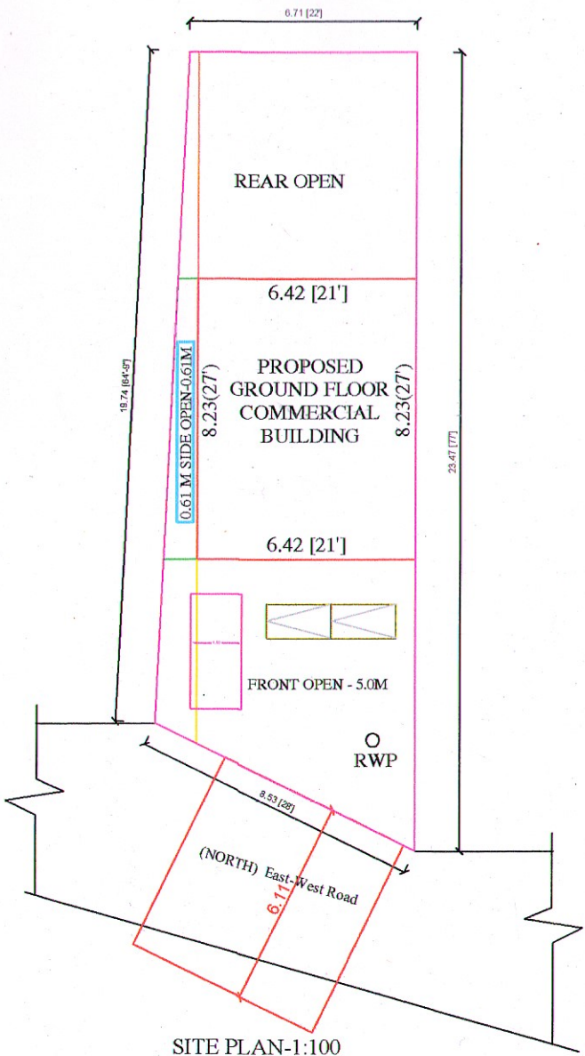
SITE PLAN-1:100
