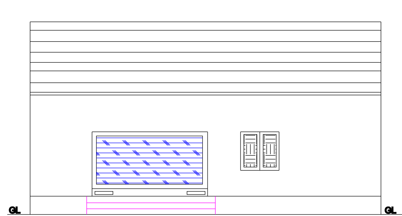
ELEVATION
