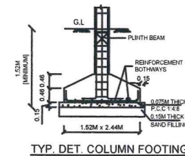
TYP. DET. COLUMN FOOTING
