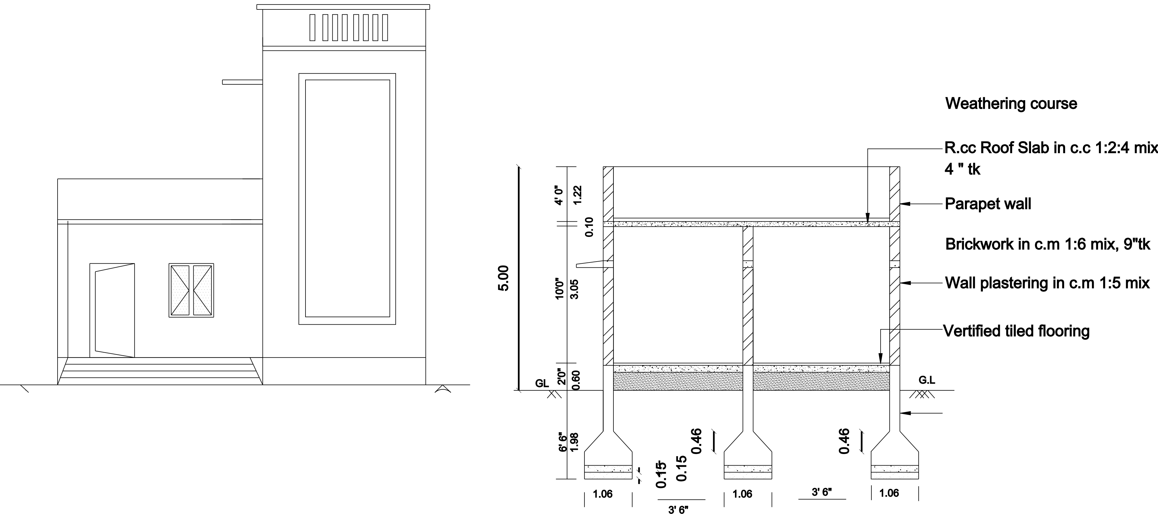
ELEVATION
