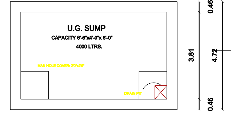
U.G. SUMP
