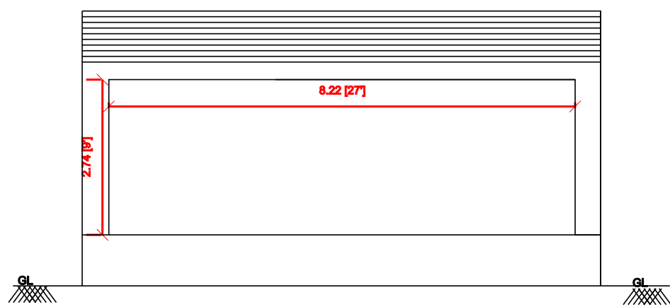
ELEVATION
