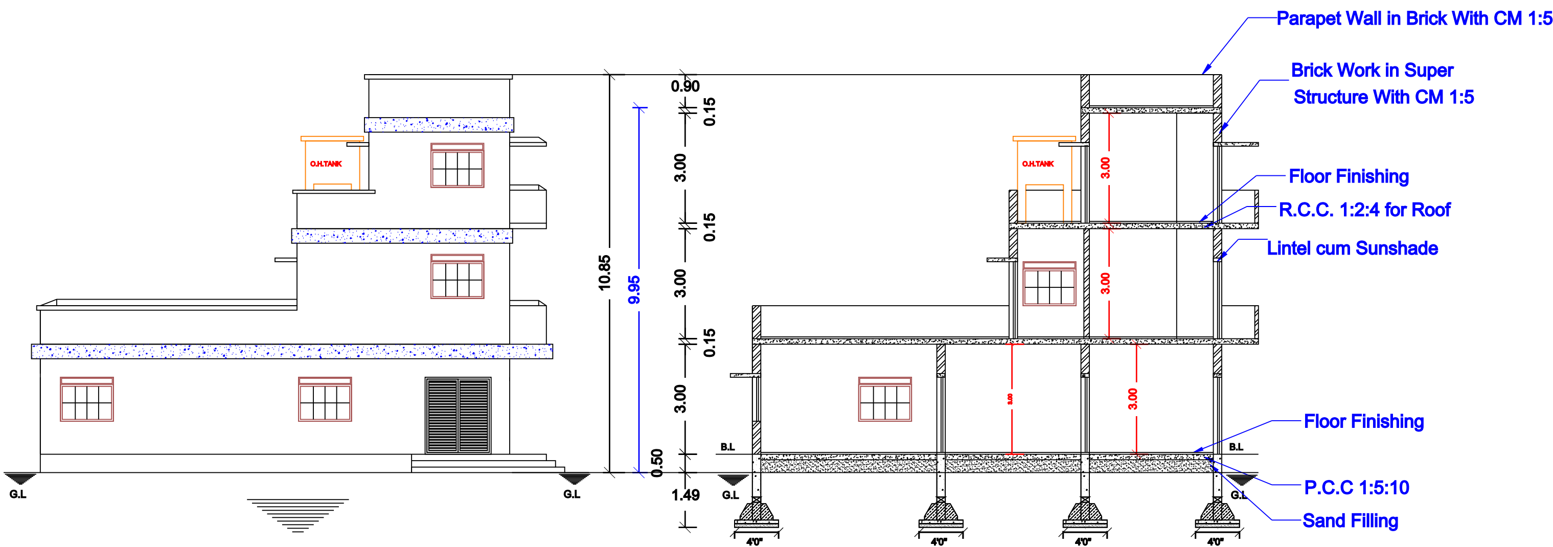
ELEVATION
