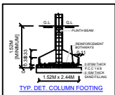
TYP. DET. COLUMN FOOTING
