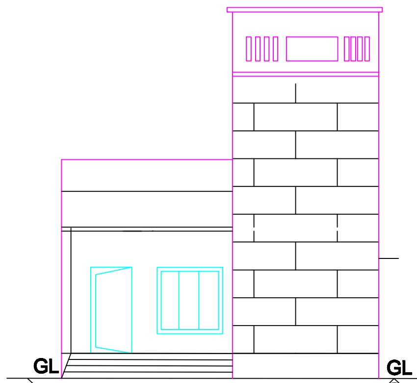
ELEVATION
