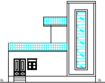
ELEVATION
