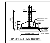
TYP DET COLUMN FOOTING
