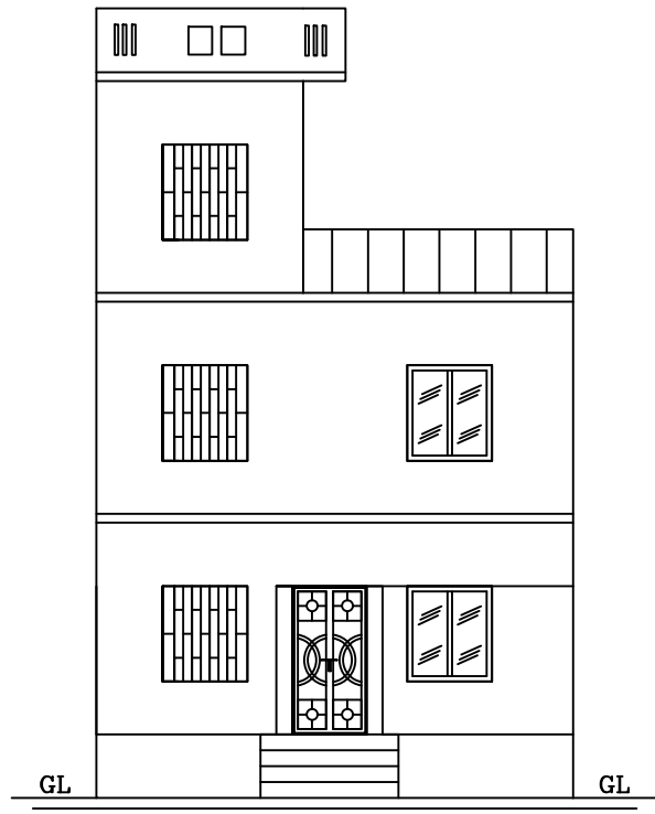
ELEVATION
