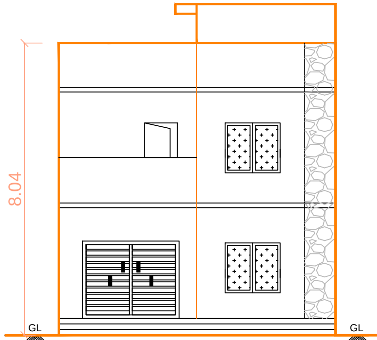
ELEVATION
