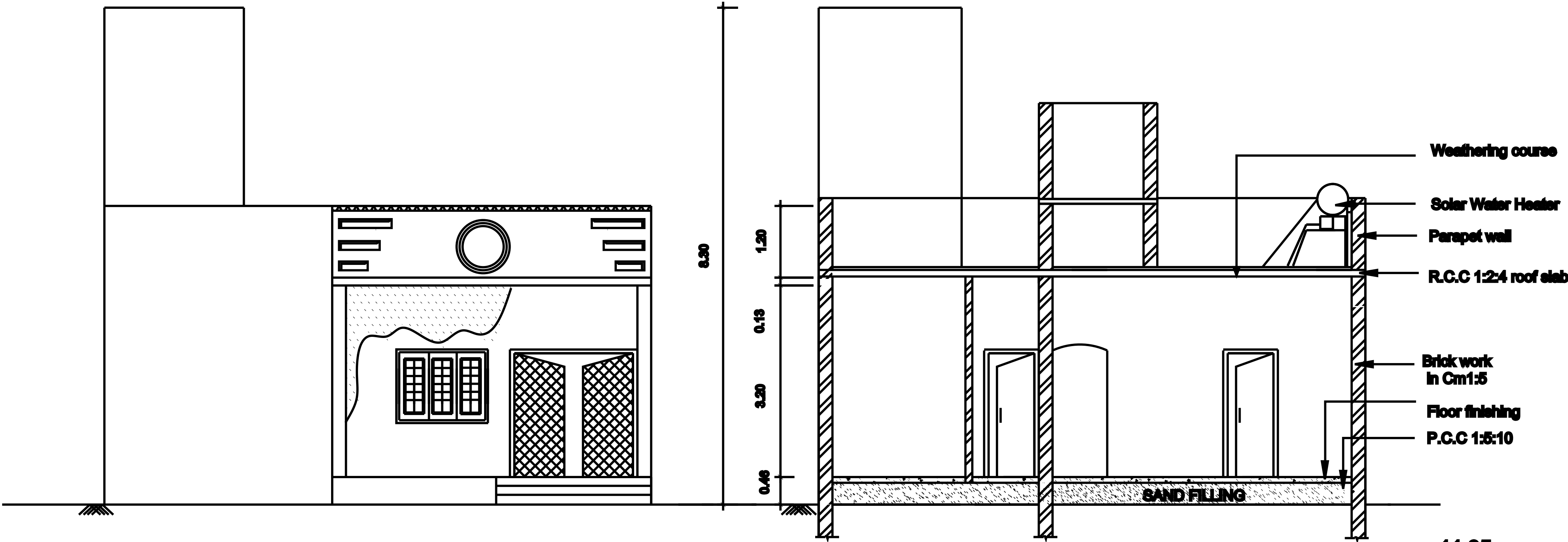
ELEVATION
